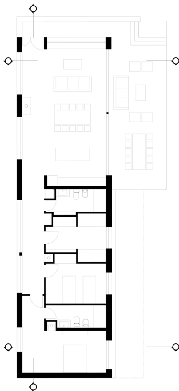
PLANTA BAJA-CASA SUR
